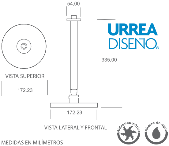
2231BT / 2231BT.9 Regadera de plato con brazo al techo Acabados: Cromo y acero inoxidable
